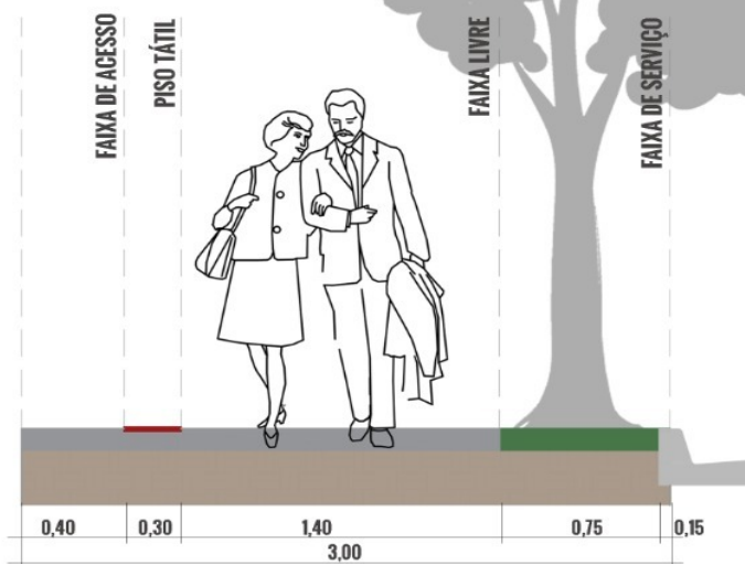
DETALHE CALÇADA
