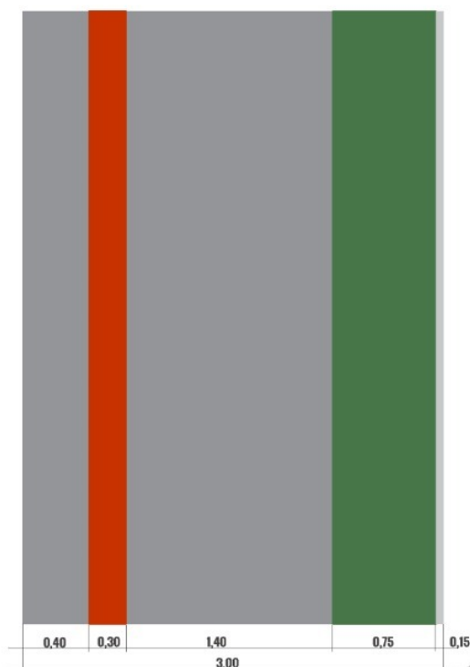
DETALHE CALÇADA
