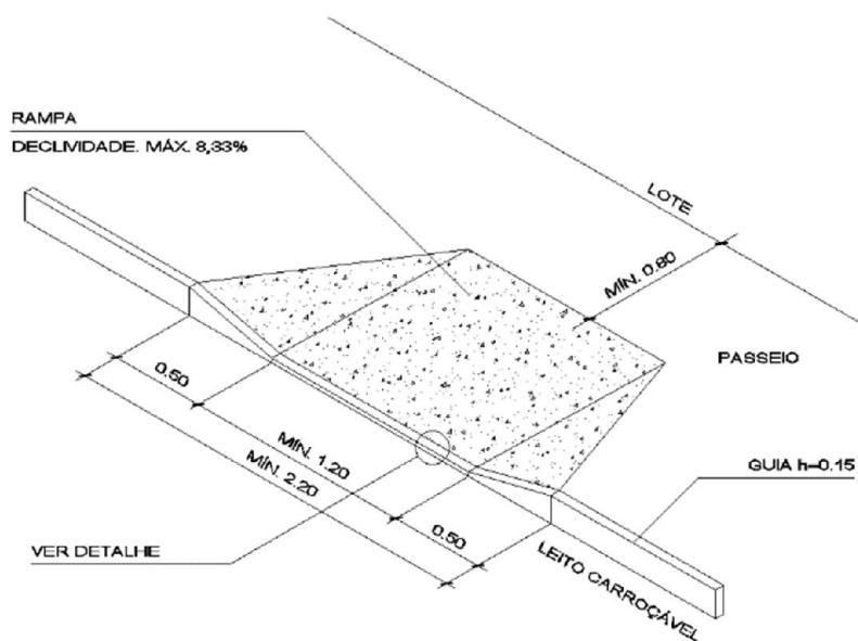
Perspectiva rampa: sem escala
