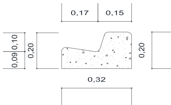
Detalhe do meio fio e sarjeta: sem escala
