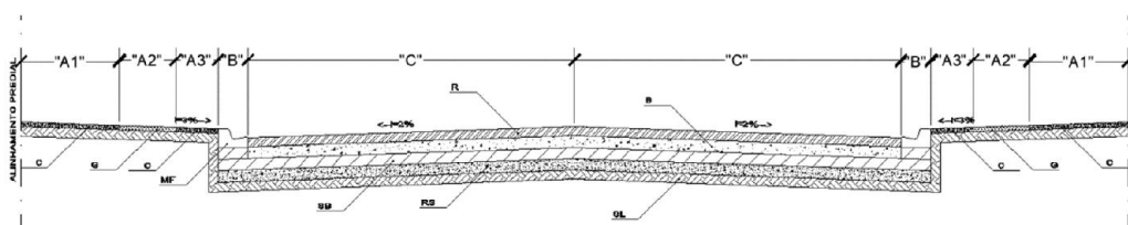
Sessão transversal de ruas e avenidas: sem escala
